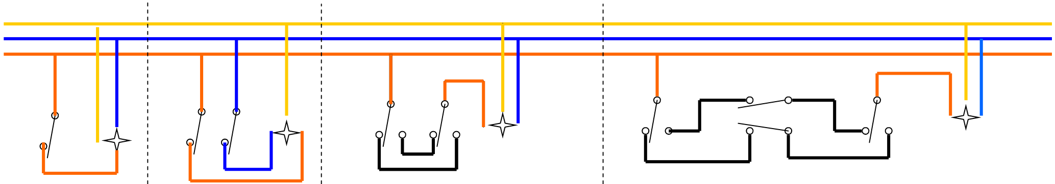
Enkelpolige kruis Schakeling
