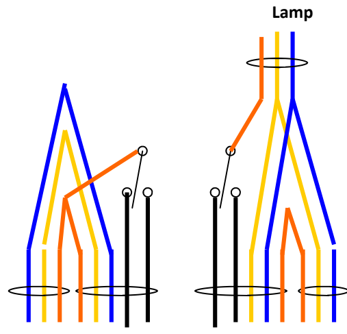
Enkelpolige Wissel Schakelaars
