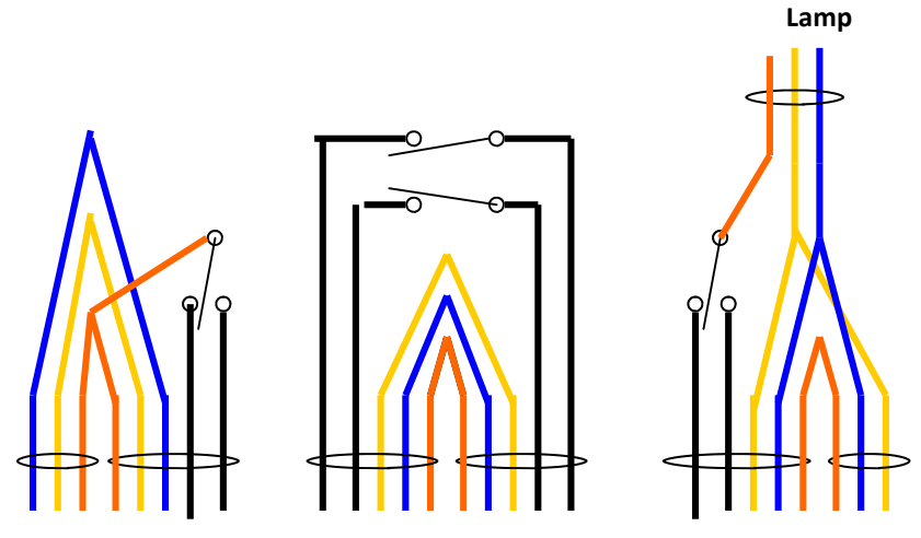
Enkelpolige kruis Schakeling
